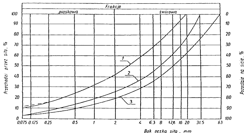
Rysunek 1. Pole dobrego uziarnienia kruszywa przeznaczonych na podbudow wykonywane metodą stabilizacji mechanicznej 1-2 kruszywo na podbudowę zasadniczą (górną warstwę) lub podbudowę jednowarstwową
